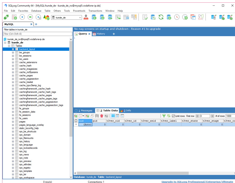
Abb. 102: SQLyog, Hauptfenster
