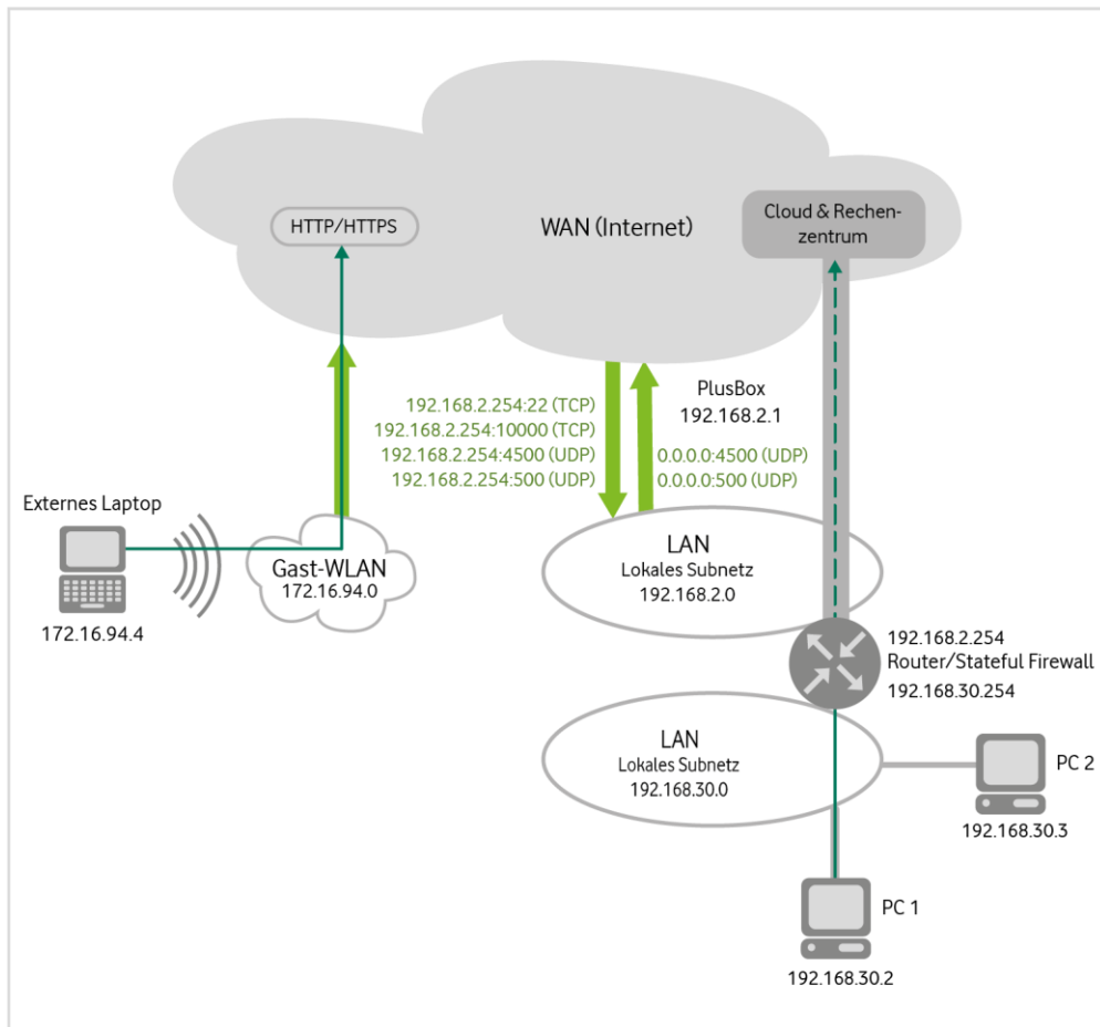
Abb. 74: PlusBox 341, Beispielkonfiguration VPN-Router im LAN
