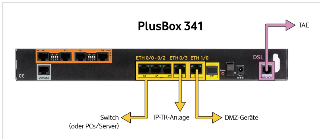
Abb. 8: Hardware-Verkabelung Anlagen-Anschluss Plus mit PlusBox 341, IP Voice + Data – Detail Autokonfig.
