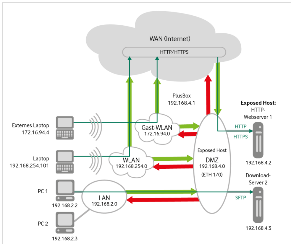
Abb. 73: PlusBox 341, Beispielkonfiguration Webserver in DMZ
