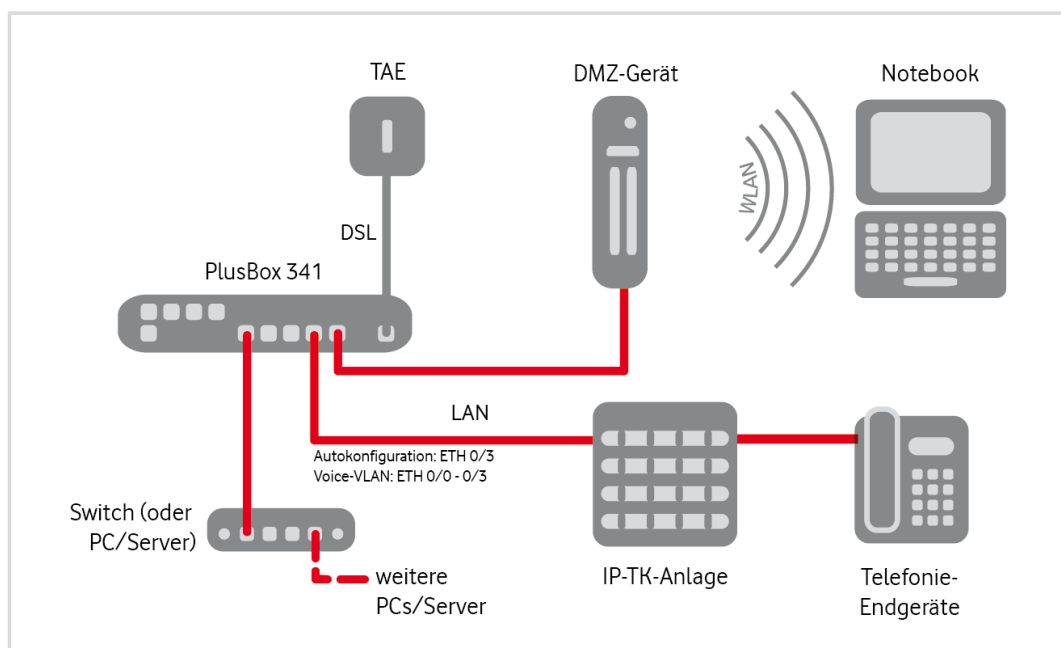
Abb. 7: Hardware-Verkabelung Anlagen-Anschluss Plus mit PlusBox 341, IP Voice + Data – Übersicht
