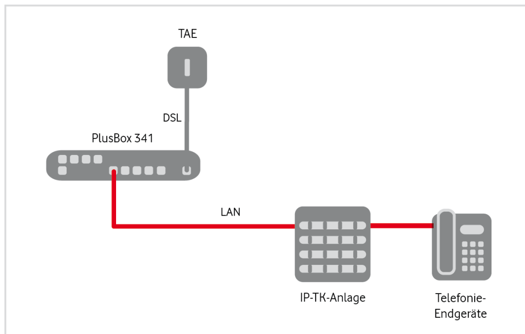
Abb. 5: Hardware-Verkabelung Anlagen-Anschluss Plus mit PlusBox 341, IP Voice only – Übersicht
