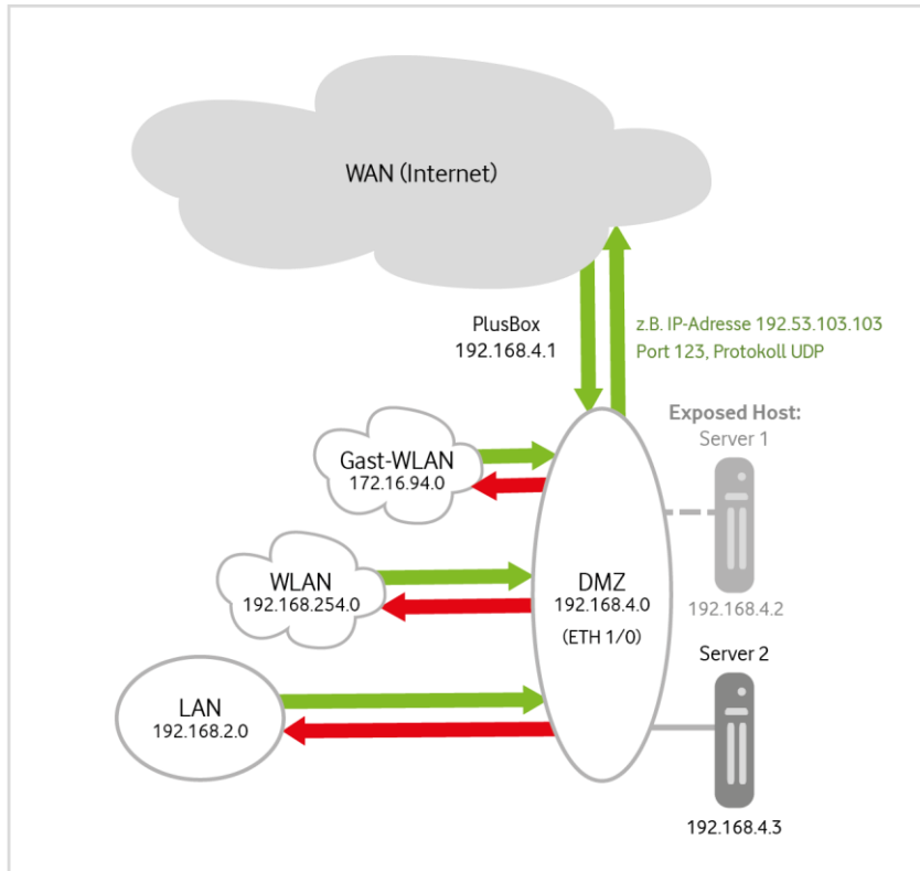
Abb. 71: PlusBox 341, Beispielkonfiguration DMZ-Rechner nutzt Internet-NTP-Server
