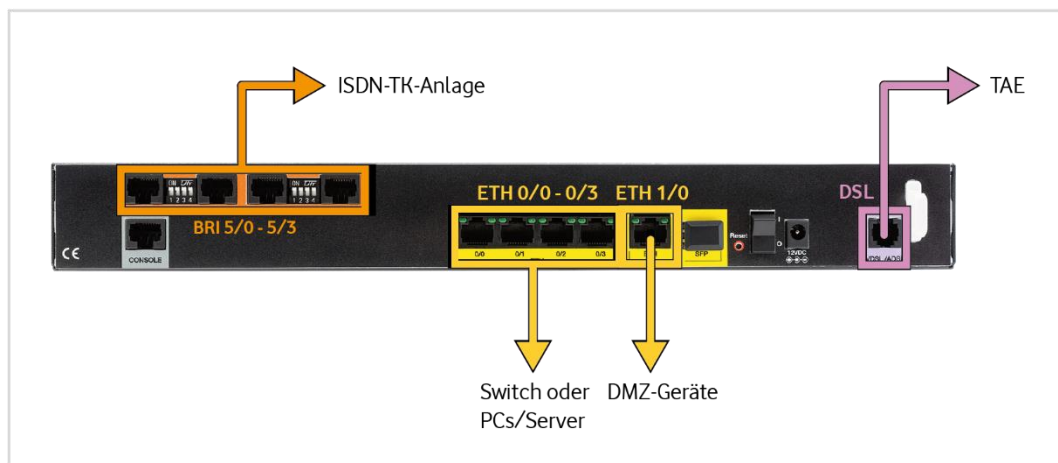
Abb. 2: Hardware-Verkabelung Anlagen-Anschluss Plus mit PlusBox 341, ISDN Voice + Data – Detail
