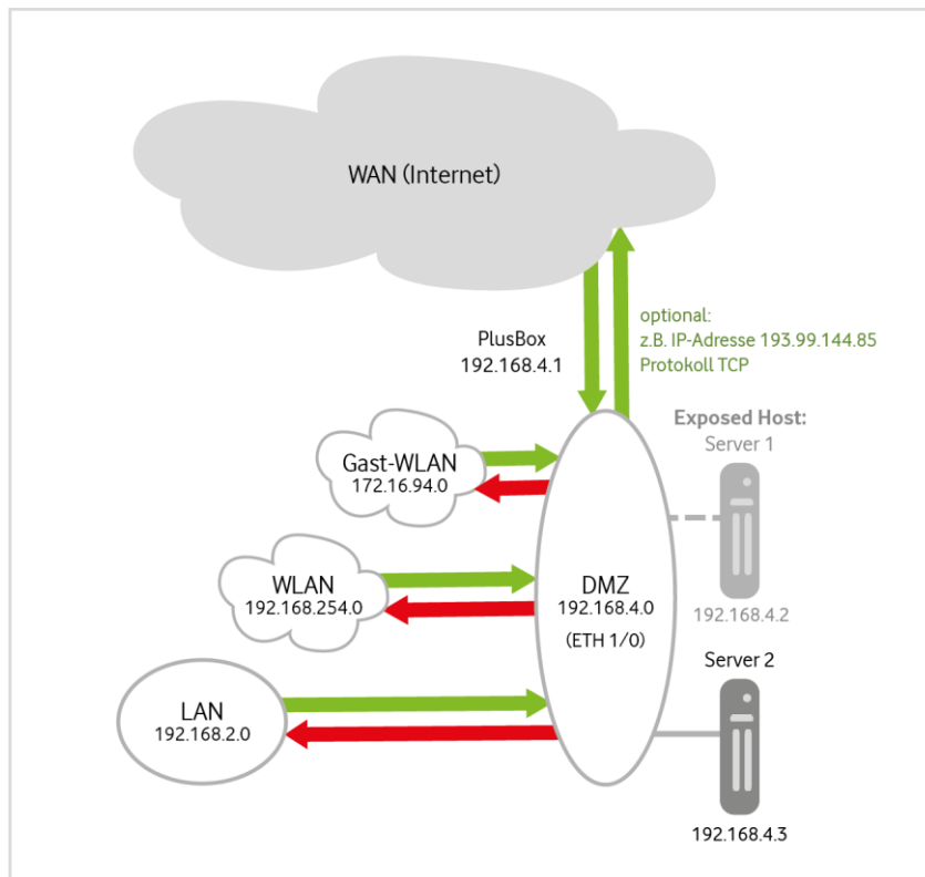
Abb. 66: PlusBox 341, Beispielkonfiguration Software-Download durch DMZ-Rechner
