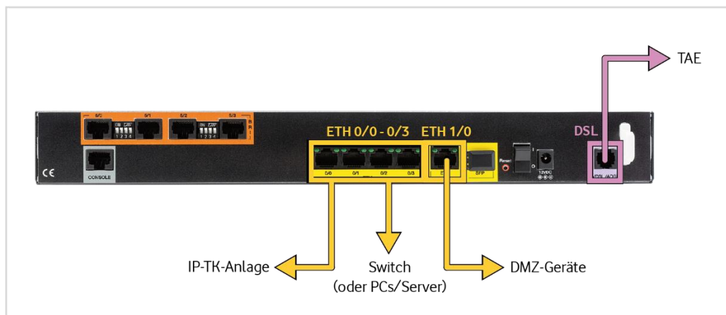
Abb. 9: Hardware-Verkabelung Anlagen-Anschluss Plus mit PlusBox 341, IP Voice + Data – Detail VLAN-Konfig.
