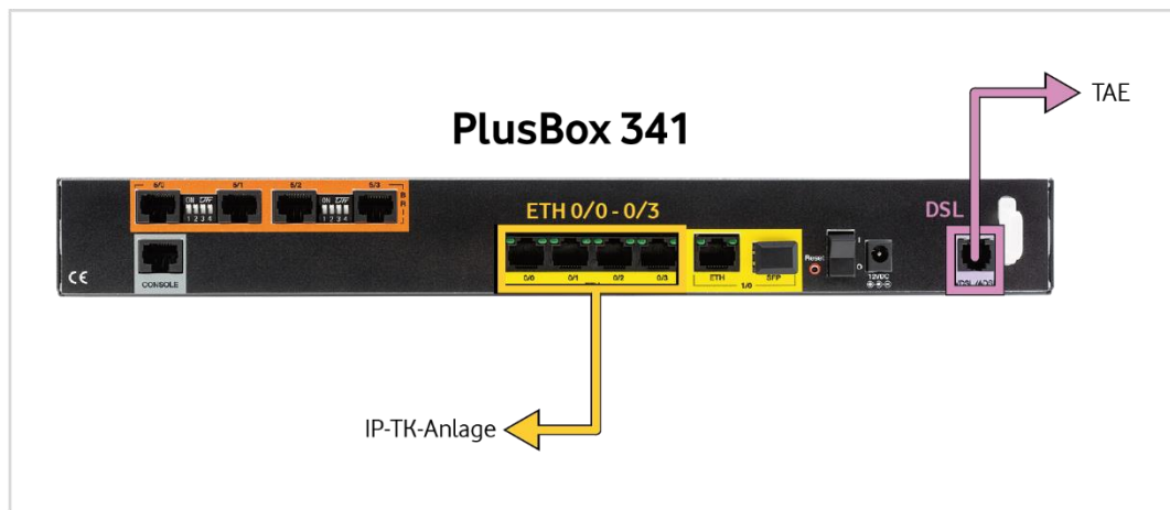
Abb. 6: Hardware-Verkabelung Anlagen-Anschluss Plus mit PlusBox 341, IP Voice only – Detail
