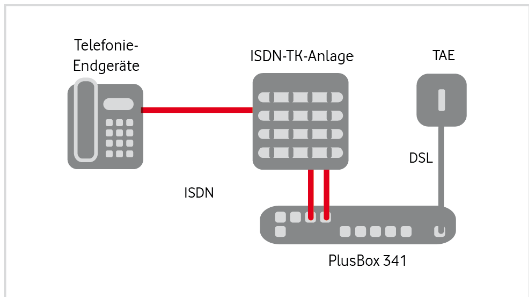
Abb. 3: Hardware-Verkabelung Anlagen-Anschluss Plus mit PlusBox 341, ISDN Voice only – Übersicht
