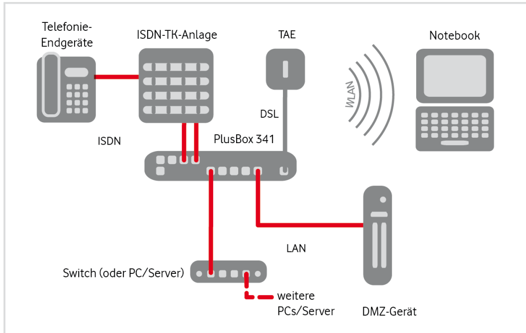
Abb. 1: Hardware-Verkabelung für Anlagen-Anschluss Plus mit PlusBox 341, ISDN Voice + Data – Übersicht
