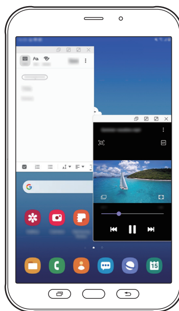
Pop-up-Ansicht
