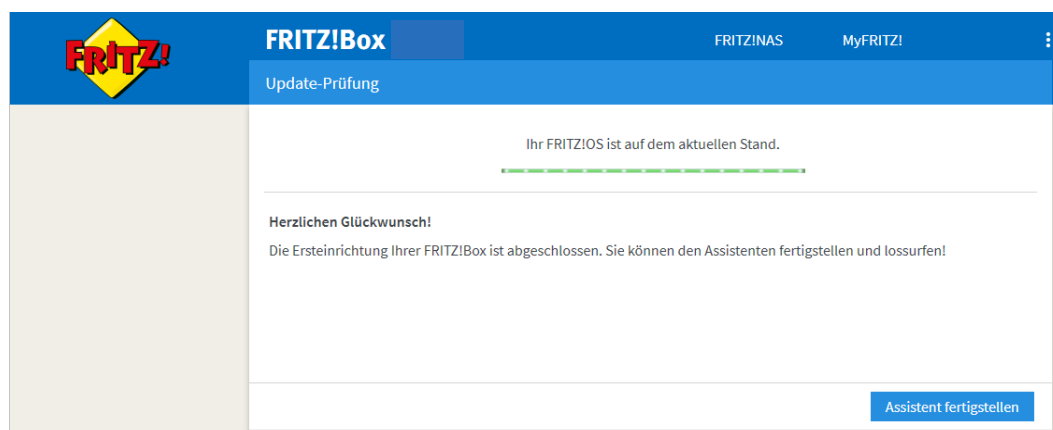
Abb. 82: FRITZ!Box, Update-Prüfung
